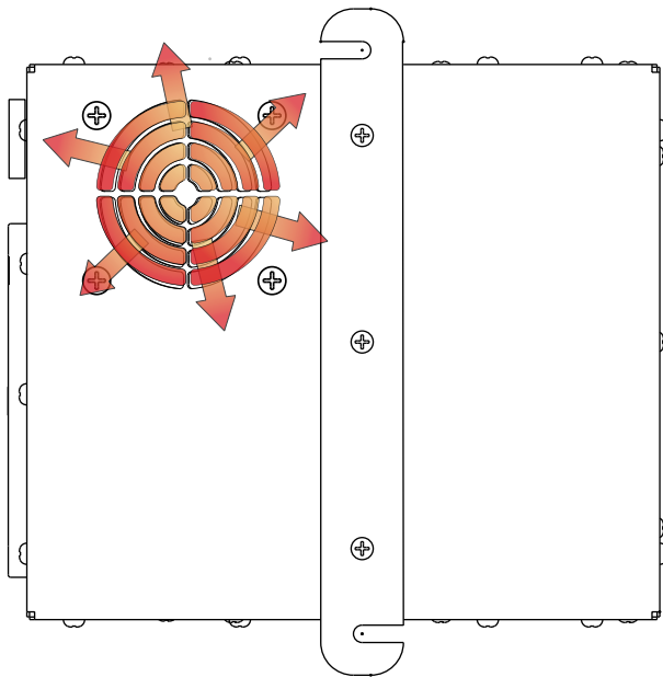
Top Outlet
